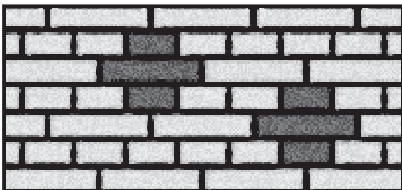
kruisverband
