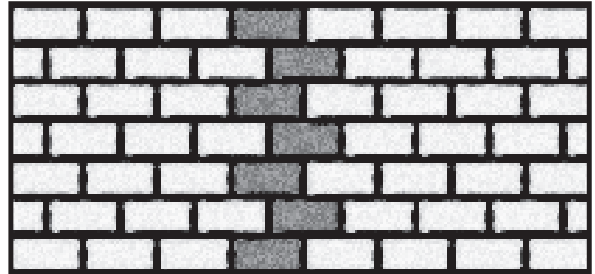
koppenverband
